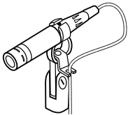
BETA 98A AN SCHWENKBAREM MIKROFONSTATIVHALTER BEFESTIGT
