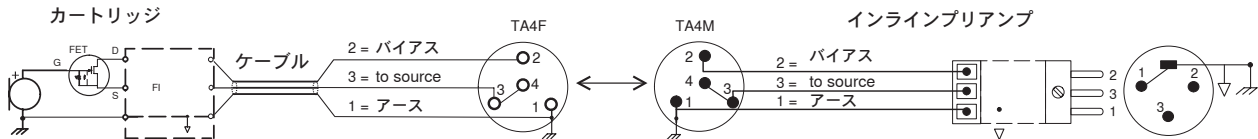
配線図
