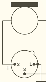
Schalt-schema U
